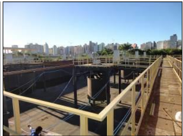
Figura 4: Reforço estrutural com cabos de aço (azul) (30/05/2014)
